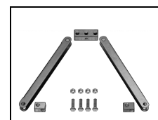
Console d'appui
