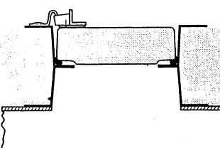
Montage à l'extérieur de la gaine (isolation épais. 50 mm)
